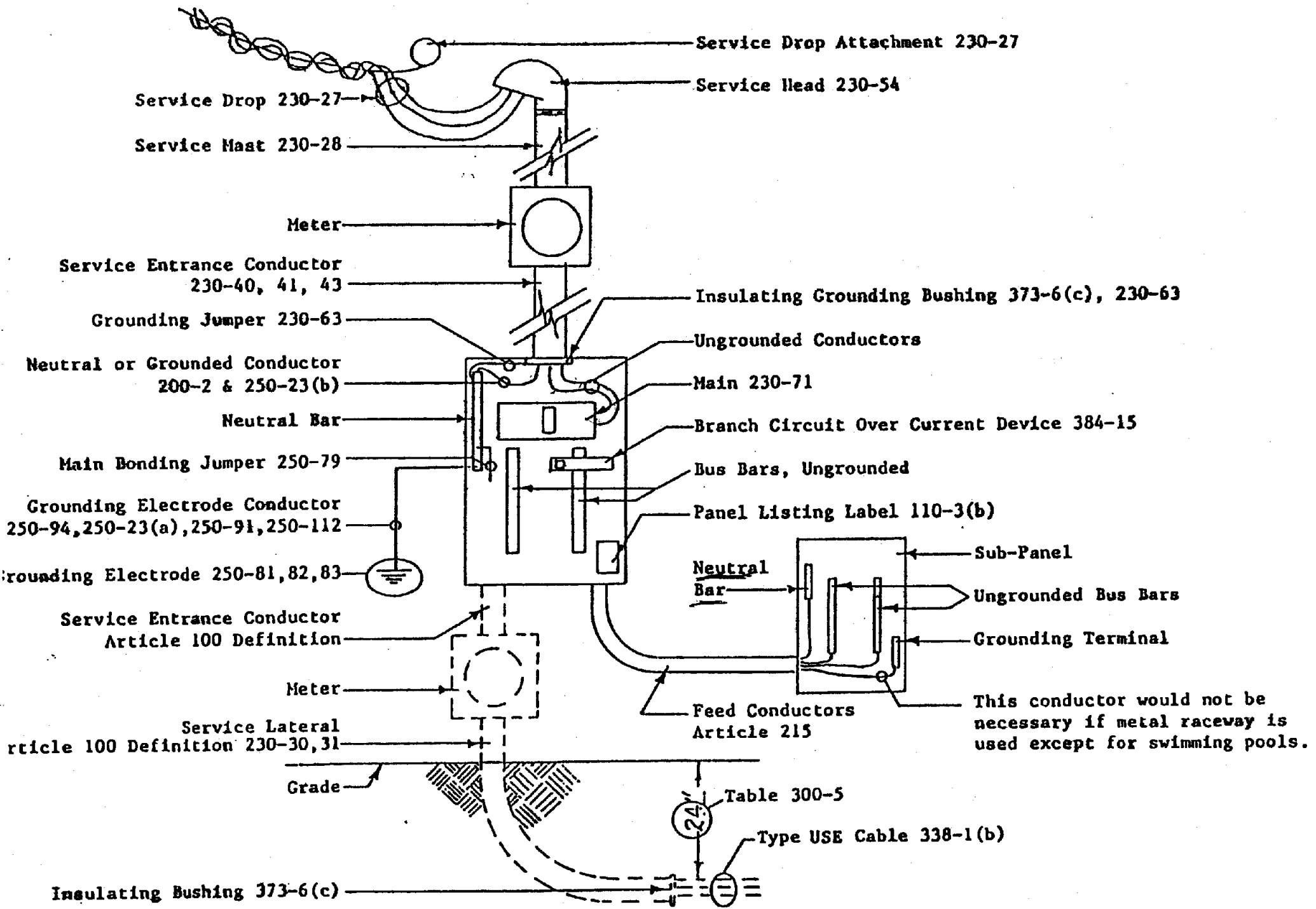
120/240 VOLT 3 WIRE 1Ø SERVICE
